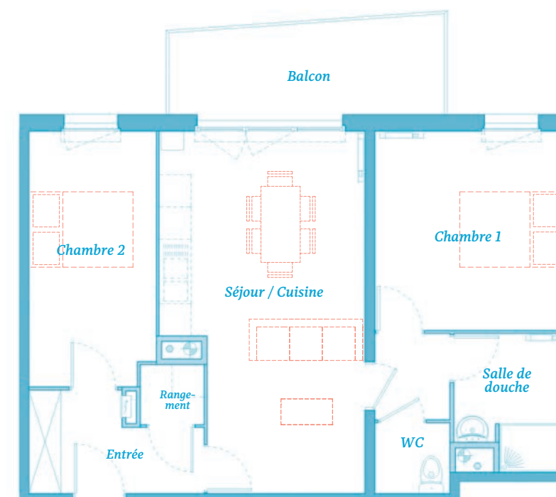
Appartement 3 pièces
