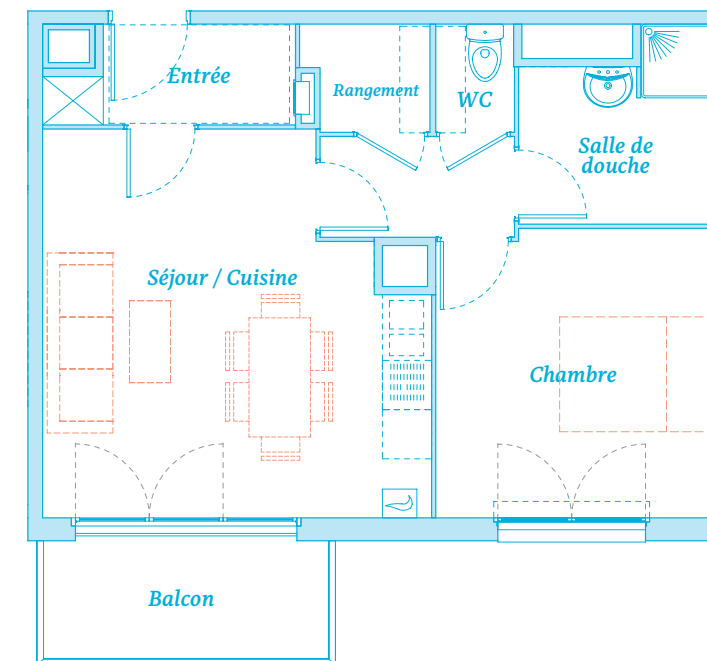
Appartement 2 pièces
