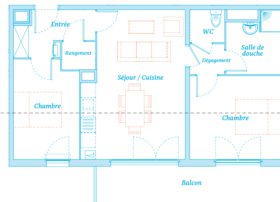
Appartement 3 pièces
